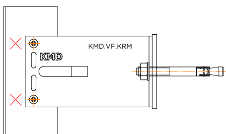
Жорстке кріплення
