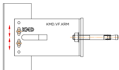
Рухоме кріплення
